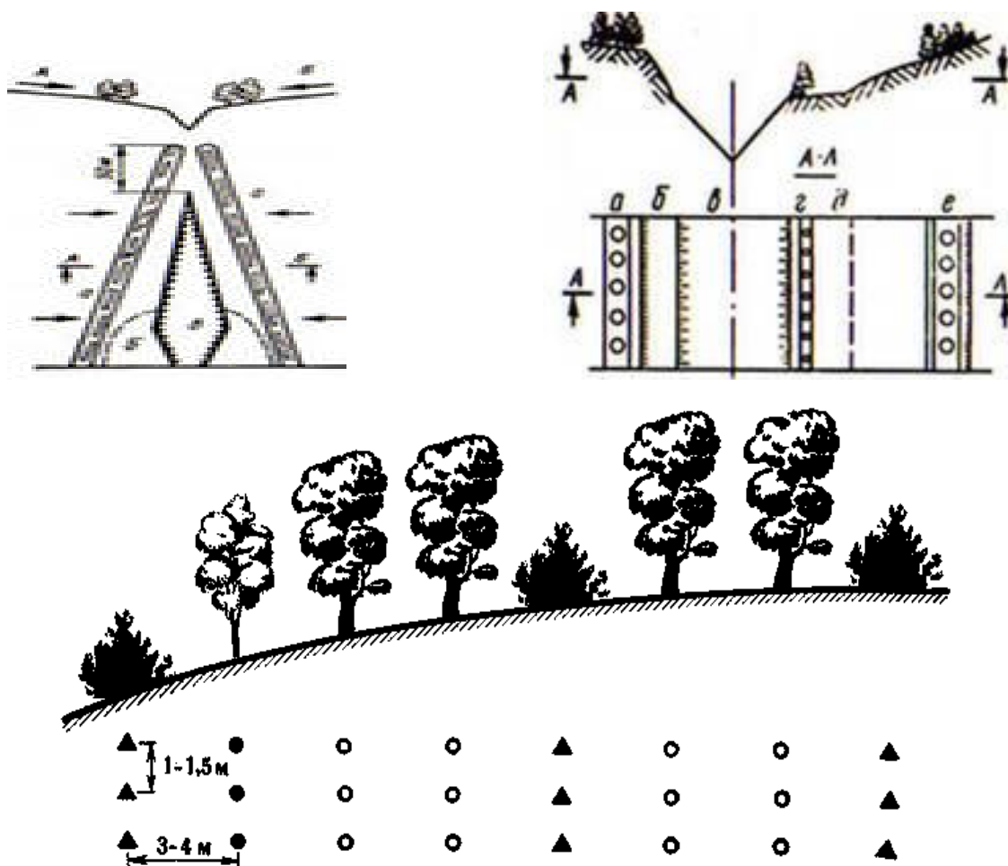
Рисунок 8 - Схема размещения приовражных лесных полос
