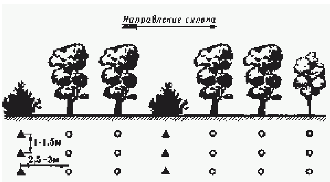
Рисунок 10 - Семирядная стокорегулирующая полоса
