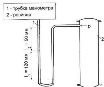
Рисунок 1.2 – Схема ресивера и манометра
