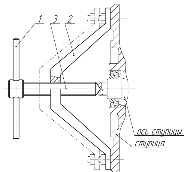
Рисунок 1.2 - Съемник И – 117.36.000
