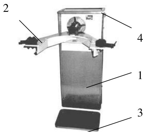
Рисунок 1.3 - Стенд для разборки и сборки двигателей Р-640: 1 – корпус; 2 – поворотный стол; 3 – поддон; 4 – пульт управления.
