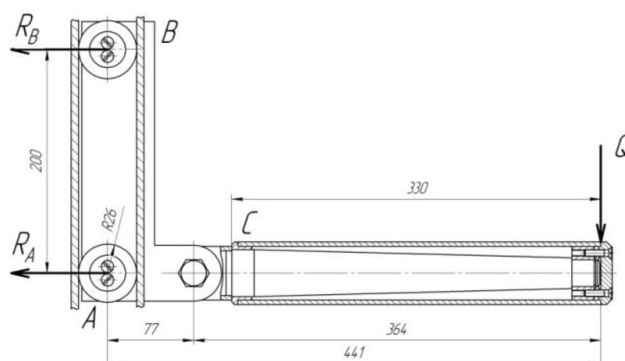
Рисунок 3.2 – Расчетная схема консоли и подвижного кронштейна Определим вес груза, действующего на консоль [2,4,7,17,18]:
