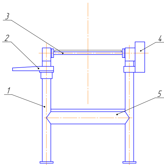
Рисунок 1.2 - Стенд для разборки и сборки двигателей Р-236: 1 – рама; 2 – полка; 3 – поворотный стол; 4 – червячный редуктор; 5 – поддон.
