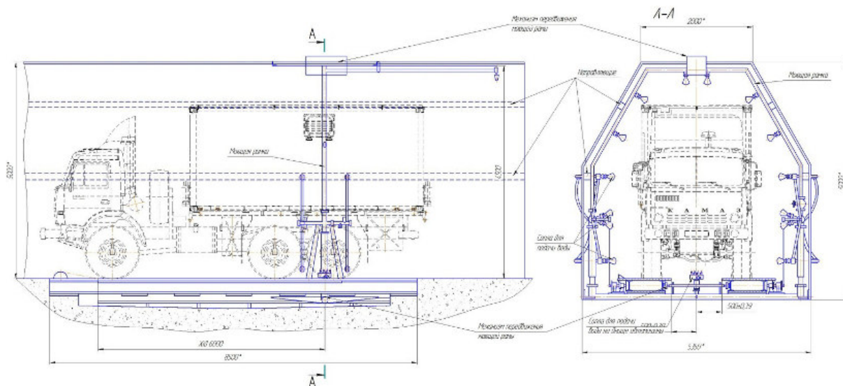
Рисунок 3.2 – Моечная установка
