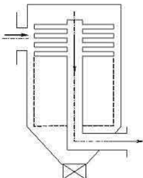
Рисунок 1.3- Схема дискового фильтра
