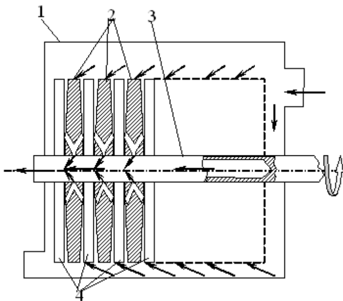
Рисунок 3.1-Схема конструкции мембранно- дискового фильтра
