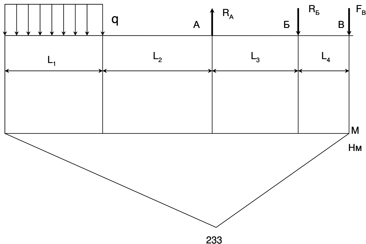
Рисунок 3.2- Эпюра изгибающих моментов вала.
