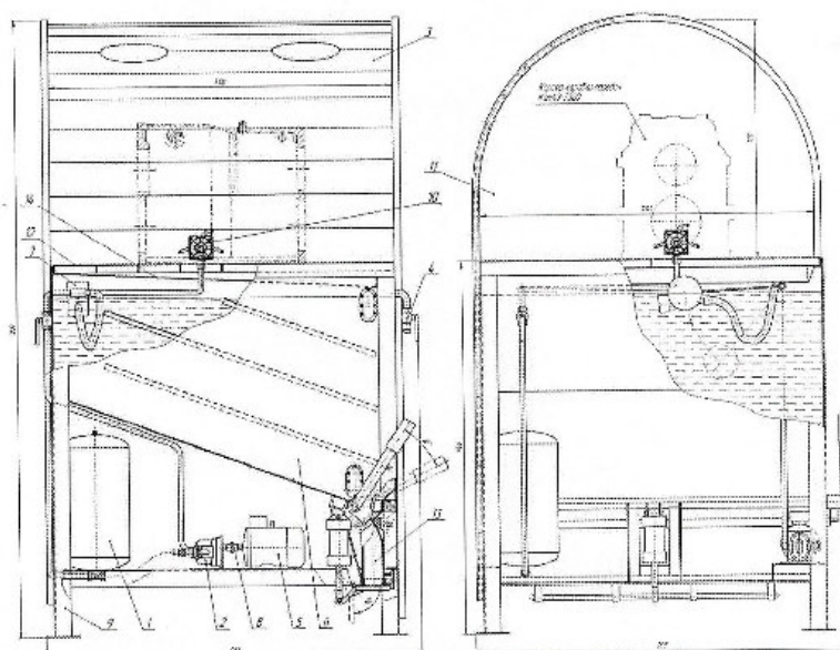
Рисунок 3.1 - Моечная установка
