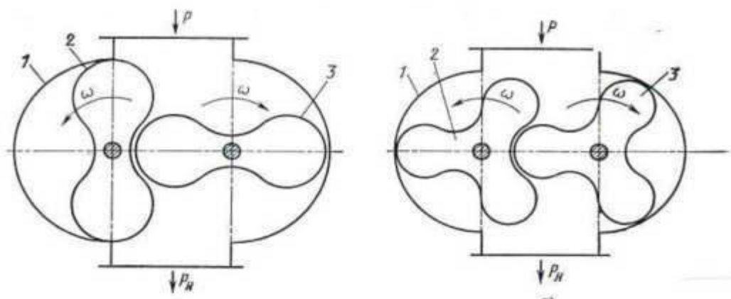
1 – корпус; 2 – ведущий ротор; 3 – ведомый ротор; P – полость всасывания; P_n – полость нагнетания Рисунок 1.6 – Схемы двухроторных насосов типа Rut's
