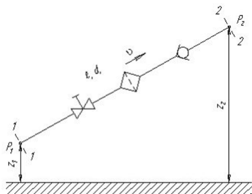
Рисунок 3.4 - Схема простого трубопровода
