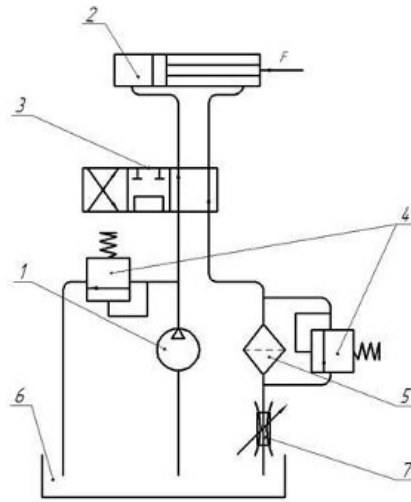
Рисунок 3.6 – Примерная схема гидропривода
