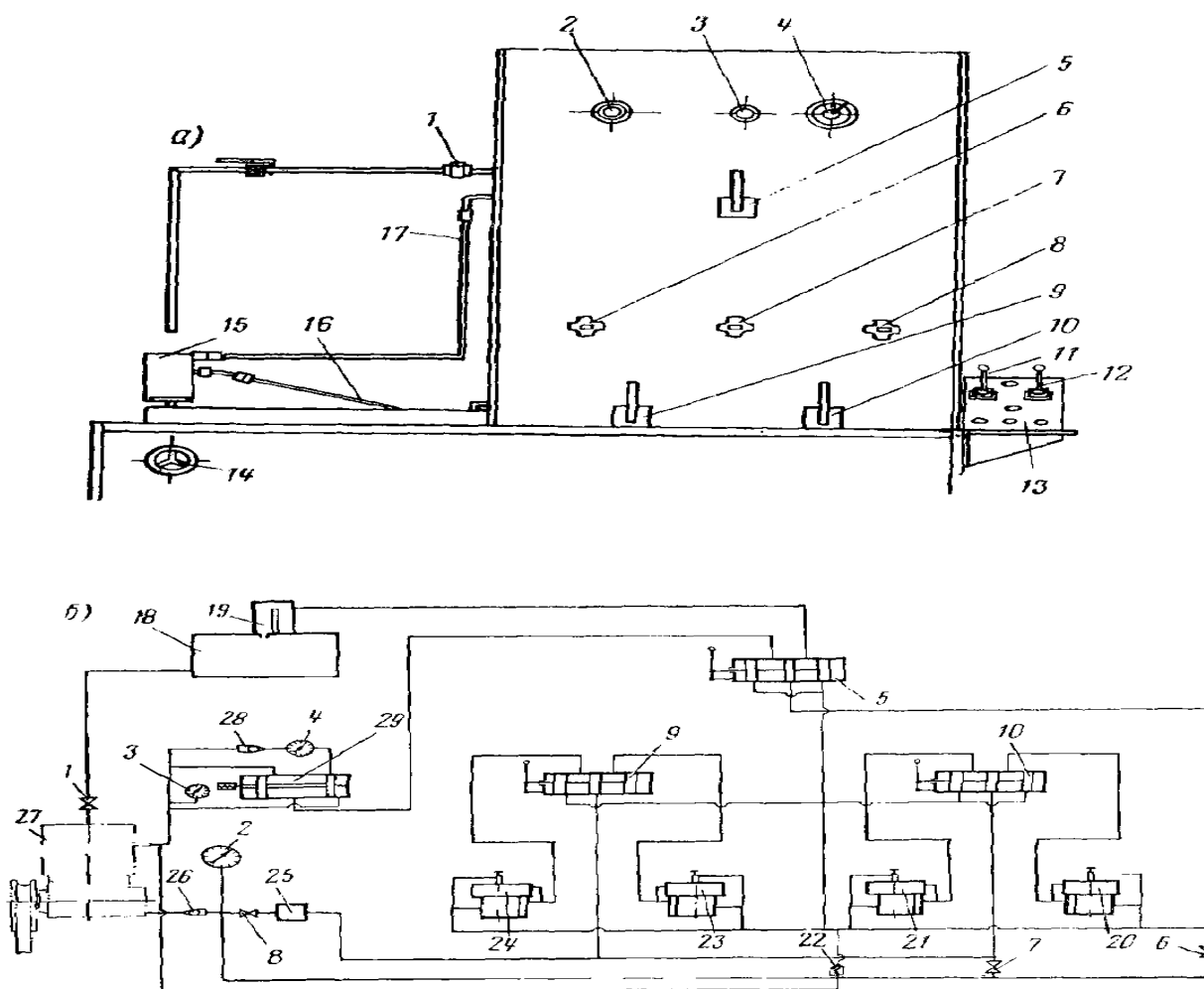
Рисунок 1 – Стенд для испытания насоса гидроусилителя рулевого управления: а — общий вид; б — гидравлическая схема.
