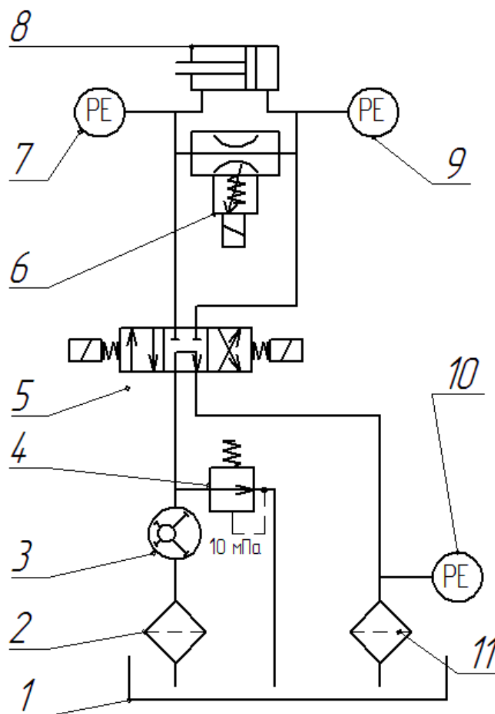
1 – гидробак; 2, 11 – фильтр; 3 – насос; 4 – предохранительный клапан; 5 – распределитель 4/3; 6 – дроссель; 7, 9 – датчики давления; 8 – нагрузатель; 10 – датчик давления сливной магистрали.
