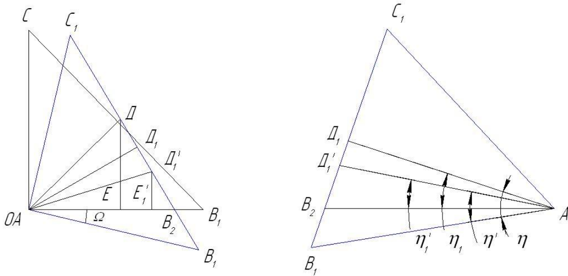
Рисунок 2.4 – Схемы для определения углов \eta'_1 и \eta_{\Gamma 1}
