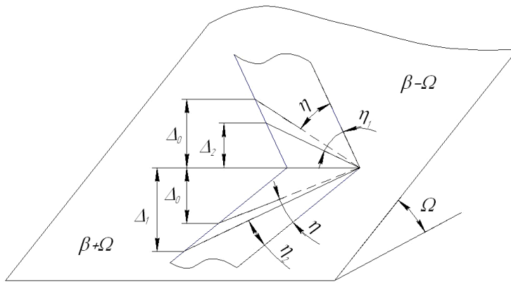
Рисунок 2.1 – Схема возникновения механической эрозии почв на склонах
