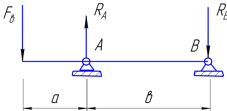
Рисунок 3.9 Балка – стык
