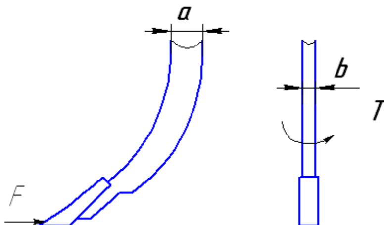
Рисунок 3.2 Расчётная схема стойки
