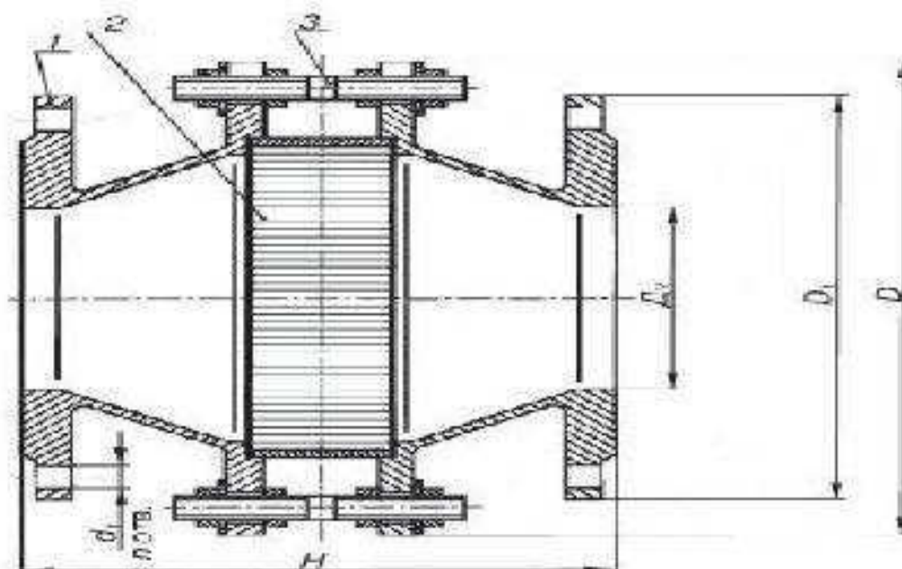
Рисунок 2.1 - Общий вид огнепреградителей ОП
