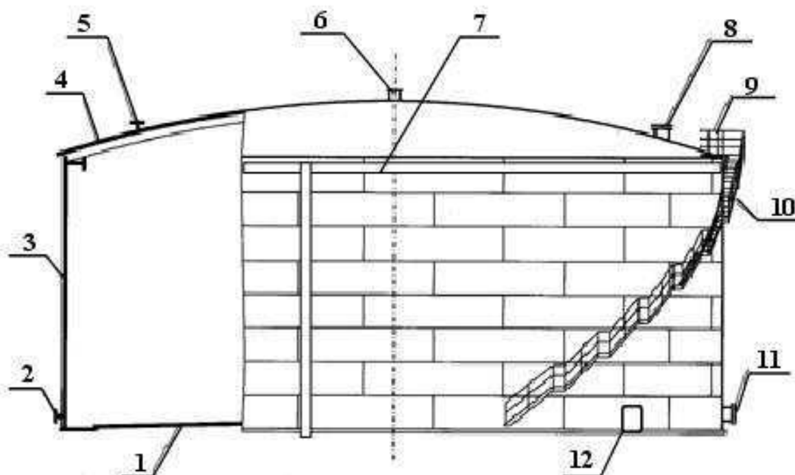
Рисунок 1.5 - Резервуар вертикальный стальной (РВС).
