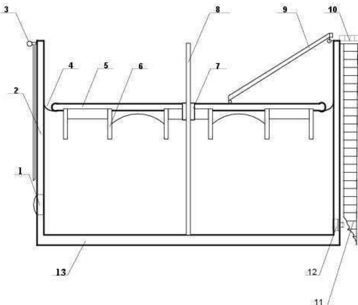
Рисунок 1.6 – Резервуар вертикальный стальной с плавающей крышей (РВСПК) 1 - люк-лаз, 2 - стенка (борт) резервуара, 3 - система охлаждения, 4 - уплотняющий затвор, 5 - плавающая крыша, 6 - опорные стойки, 7 - затвор-кожух, 8 - вертикальная направляющая, 9 - лестница с поворотным устройством, 10 - смотровая площадка, 11 - стационарная лестница, 12 - сливно-наливная арматура, 13 - днище резервуара жидкости, для предотвращения их выхода из под понтона служит периферийная юбка
