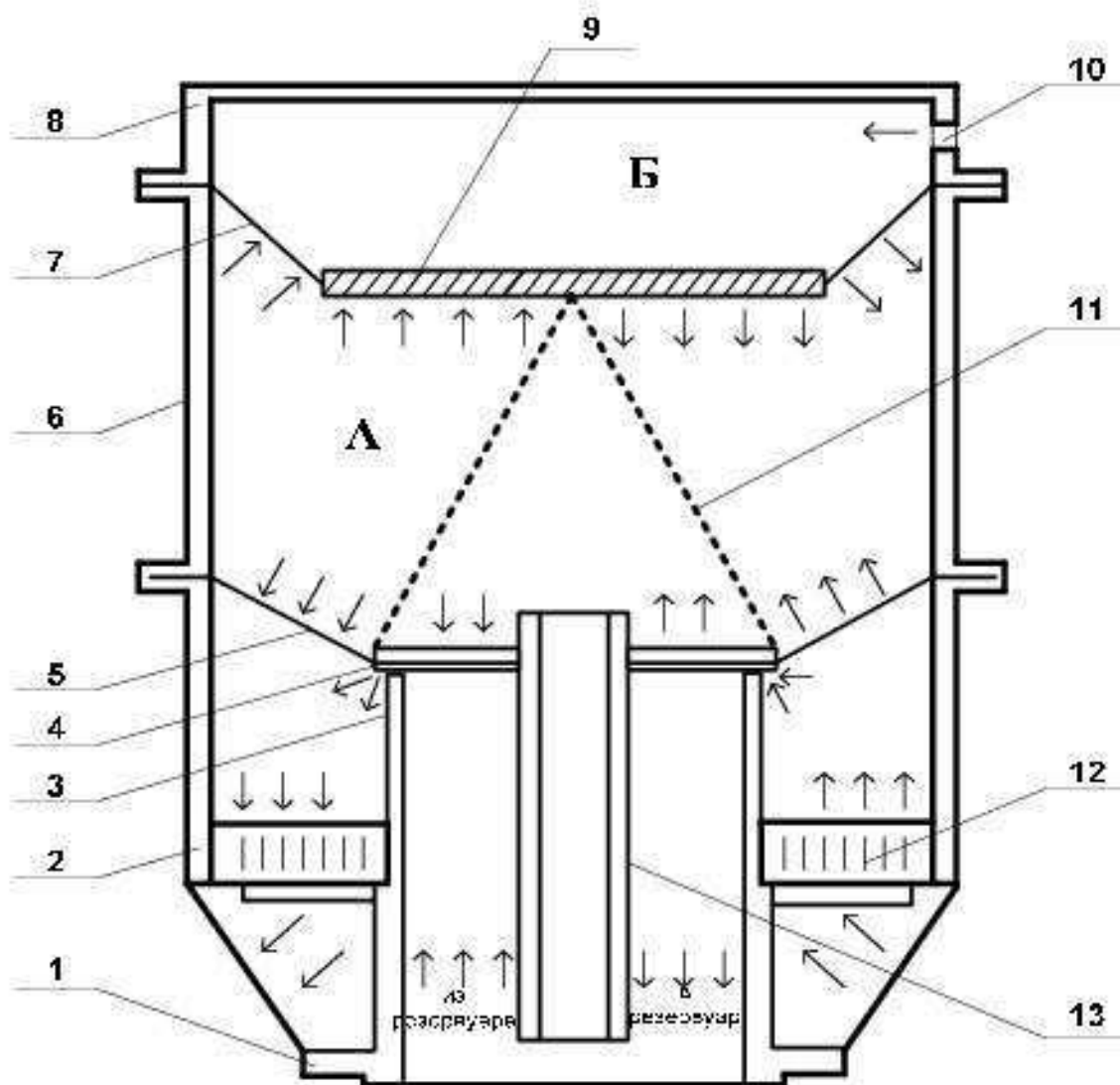
Рисунок 1.9 - Немерзающий дыхательный клапан типа НДКМ
