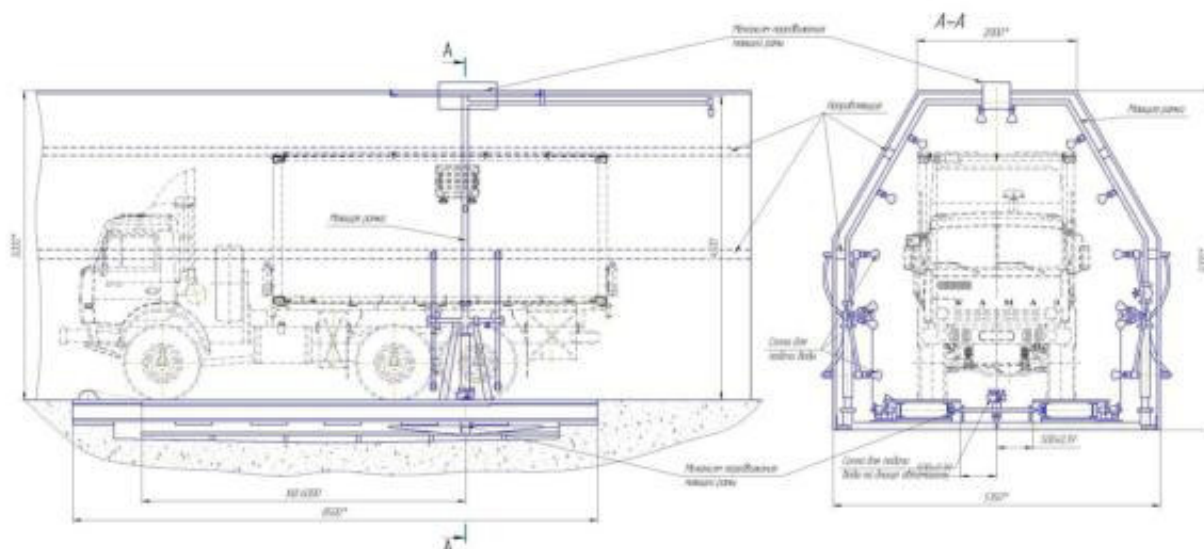
Рисунок 3.2 – Моечная установка
