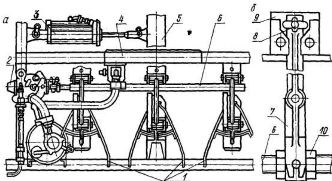
Рисунок 3 – Автомат вождения
