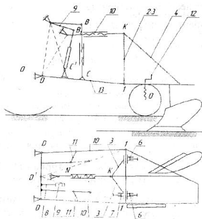
Рисунок 4.8 - Схема навешивания плуга на трактор
