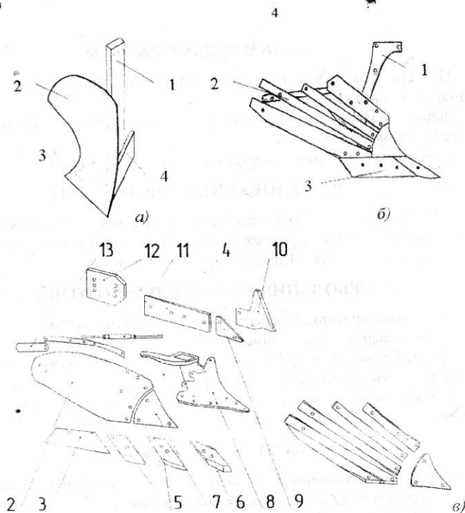
1 – стойка; 2 – отвал; 3 – лемех; 4 – полевая доска; 5 – острый лемеха; 6 – привинчиваемое острие; 7 – кромка отвала; 8 – башиак корпуса; 9 – клин полевой доски; 10 – нож полевой доски; 11 – опора отвала; 12 – защита полевой доски; 13 – удлинитель отвала Рисунок 4.1 – Корпуса для отвальной вспашки а) корпус обычный; б) корпус с пластинчатым «перьевым» отвалом; в) основные узлы корпусов плугов
