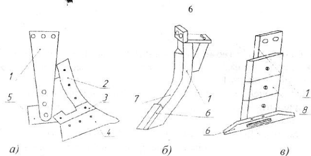
а) 1 – стойка; 2 – щиток; 3 – упоритель лемеха; 4 – лемех; 5 – полевая доска; б) 6 – долото; 7 – обтекатель; 8 – нож Рисунок 4.3 – Корпуса плугов для безотвальной вспашки: а) корпус Мальцева, б) чизельный плуг; в) корпус «Параплан»
