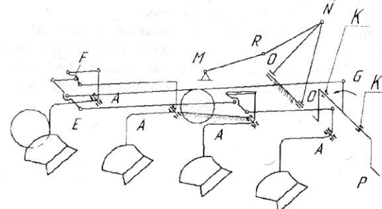
Рисунок 4.10 - Схема плуга ПКС - 4-35
