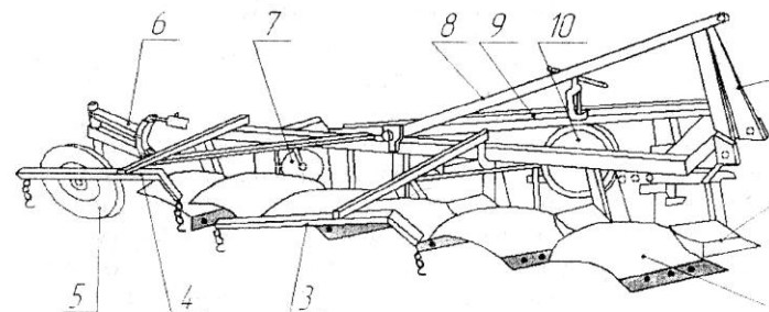
Рисунок 4.5 - Плуг ПЛП-6-35
