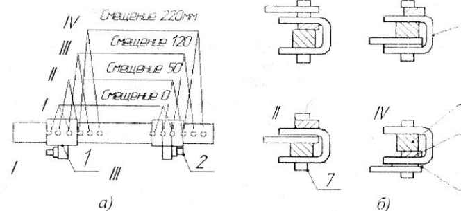
Рисунок 4.6 - Схемы установки: а) кронштейнов на поперечной балке; б) штока догрузителя
