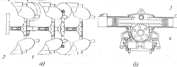
1 - рама плуга; 2 - оборотный механизм; 3 - рейка механизма; 4 - шестерня
