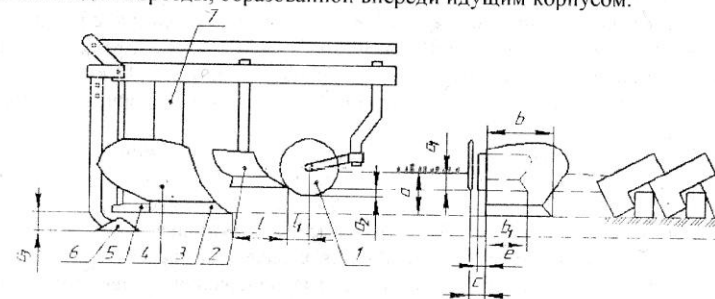
1 – дисковый нож, 2 – предплужник, 3 – лемех, 4 – отвал, 5 – полевая доска, 6 – почвоуглубитель
