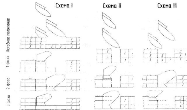
Рисунок 4.12 - Схемы перемещения пластов почвы плугом ПТН-40
