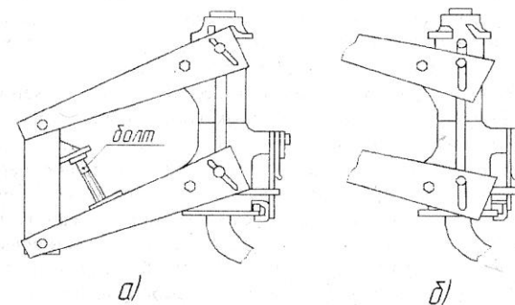
Рисунок 4.7 - Механизм заднего колеса: а) рабочее положение, б) транспортное положение
