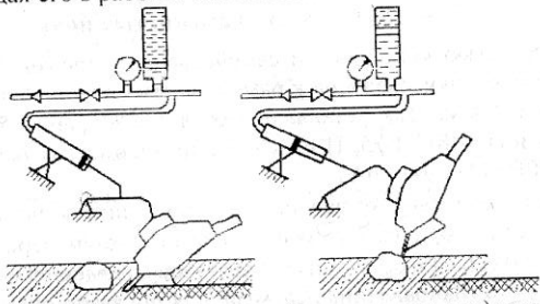
Рисунок 4.11 - Схема работы пневмогидравлического предохранительного механизма
