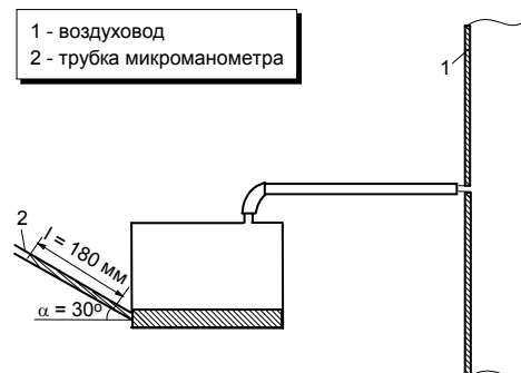
Рисунок 1.1 – Схема воздуховода и микроанометра
