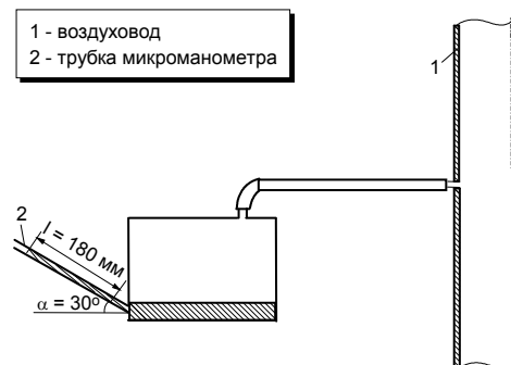
Рисунок 1.1 – Схема воздушовода и микроманометра
