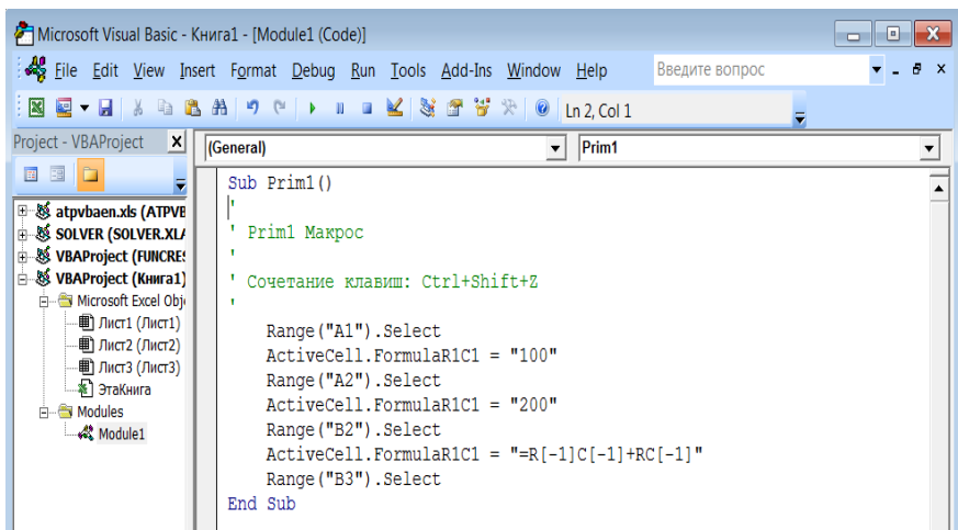
Рис. 1.3. Окно редактора VBA.
