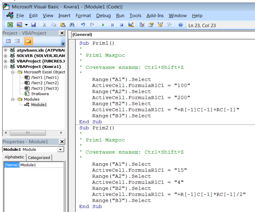
Рис. 1.4. Окно редактора VBA.
