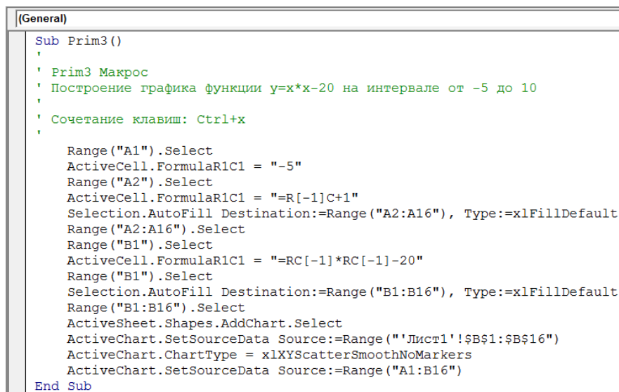
Рис. 1.7. Код инструкций макроса.
