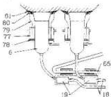
Рисунок 3.1 - Автоматизированная мобильная доильная установка
