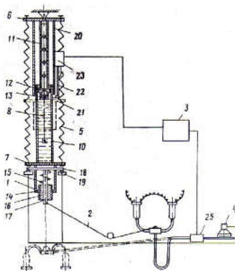
Рисунок 1.6 - Схема устройства для снятия донльного аппарата
