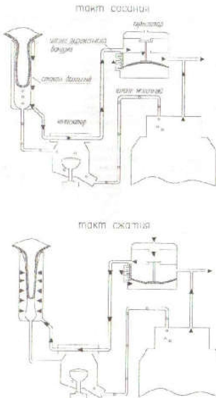
Рисунок 1.5 – Схема работы аппарата доньного
