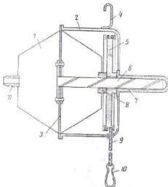
Рисунок 1.8 - Устройство для снятия донльных аппаратов.
