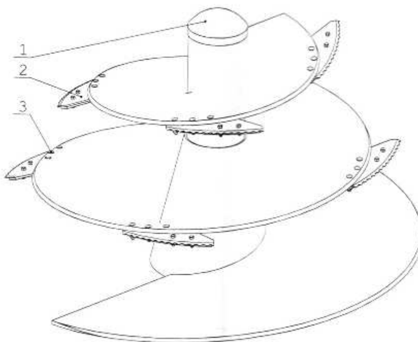
Рисунок 1.6 – Шнек
