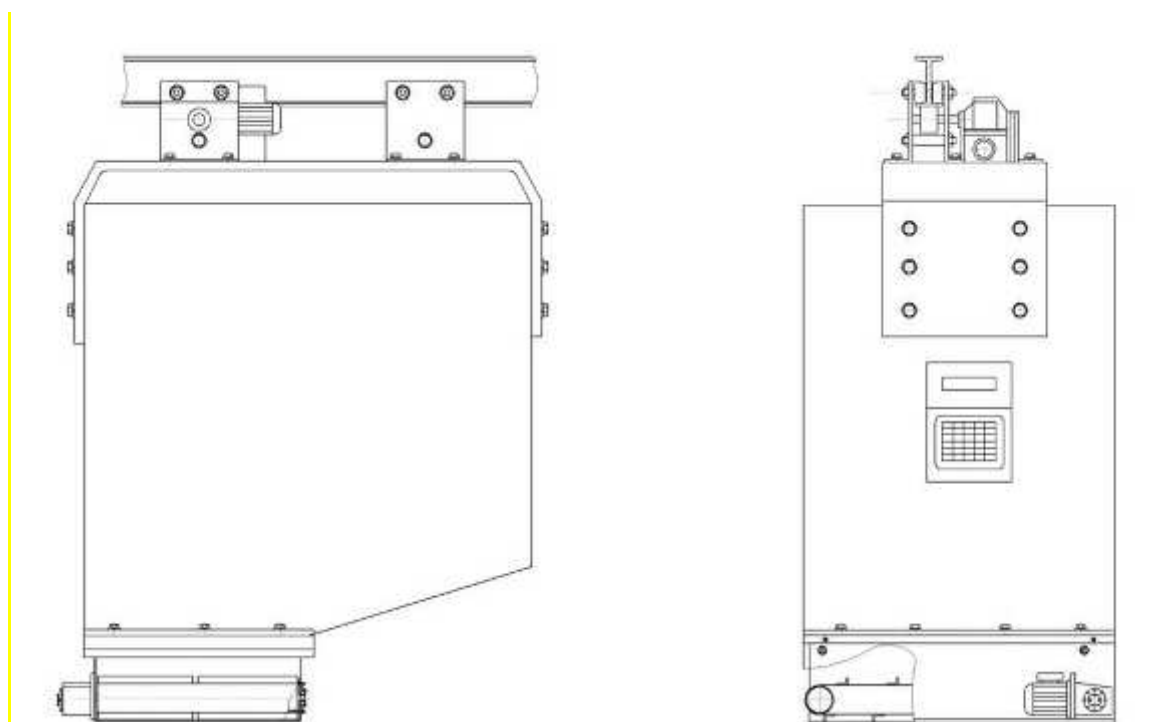
Рисунок 3.1 – Схема разрабатываемого мобильный кормораздатчик
