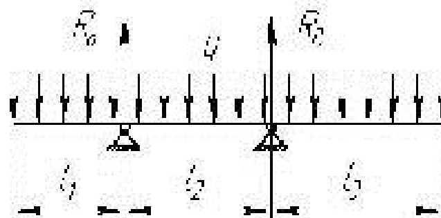
Рисунок 3.1 – Схема действия сил
