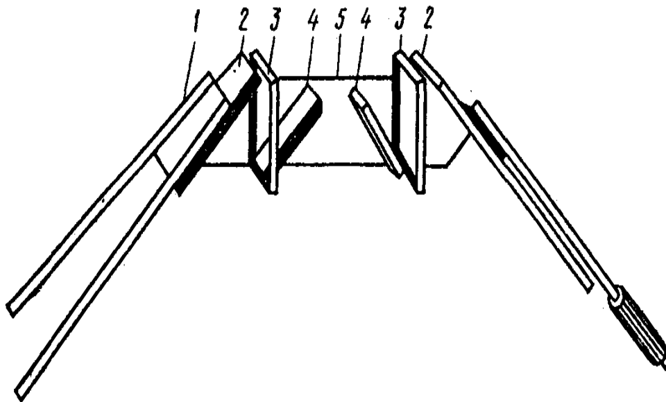
Рис.1 Линзово-зеркальный стереоскоп:
