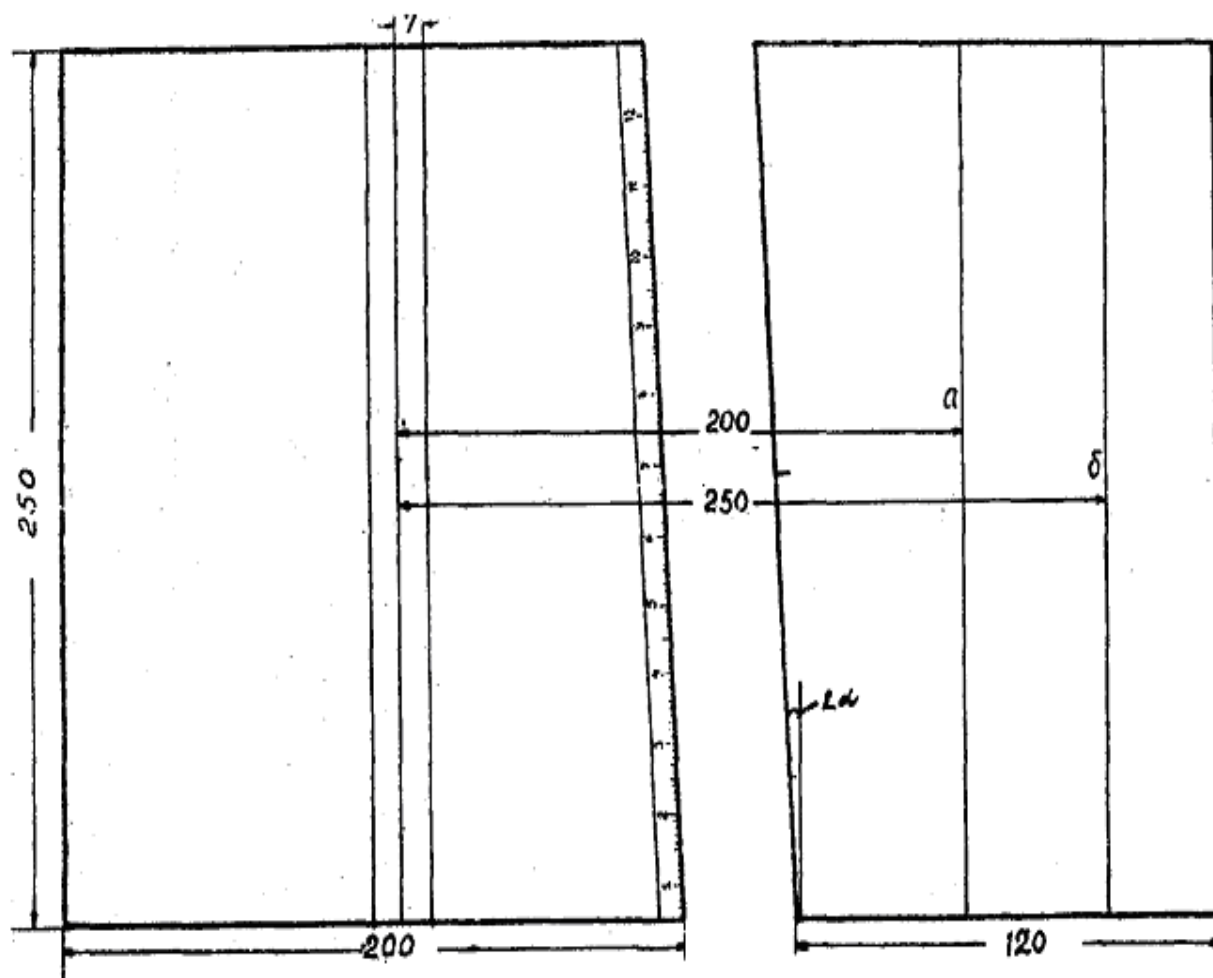
Рис.12 Параллактические пластины
