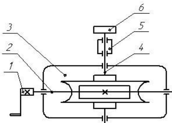
Рисунок 3.1 - Кинематическая схема стенда
