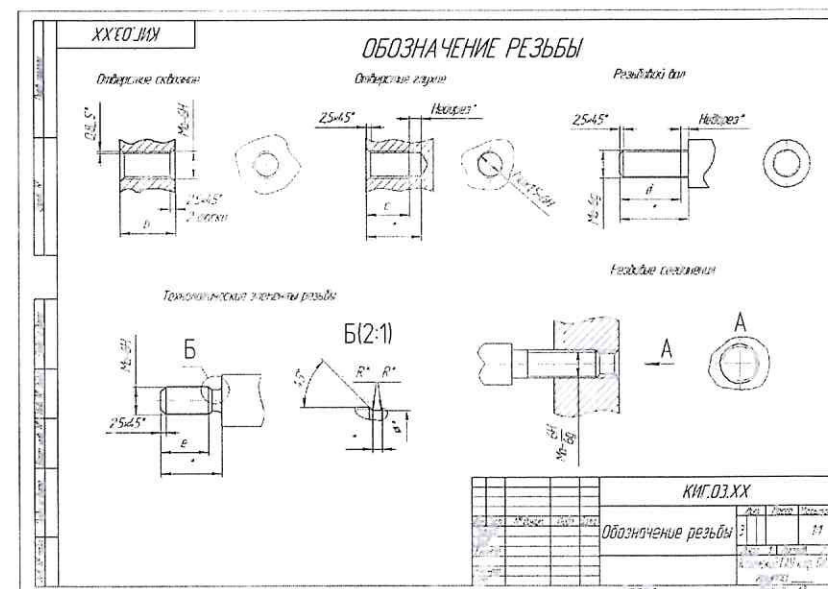
Задание 3. Выполнить чертежи резьбовых элементов и соединений.
