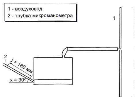
Рисунок 1.1 – Схема воздуховода и микроманометра
