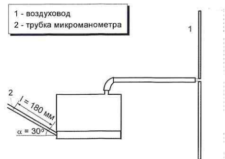
Рисунок 1.1 – Схема воздушовода и микроманометра
