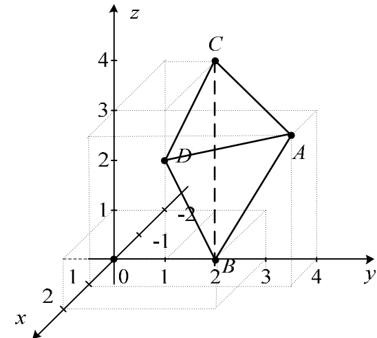
Рисунок 4 – Пирамида ABCD в пространстве XYZ
