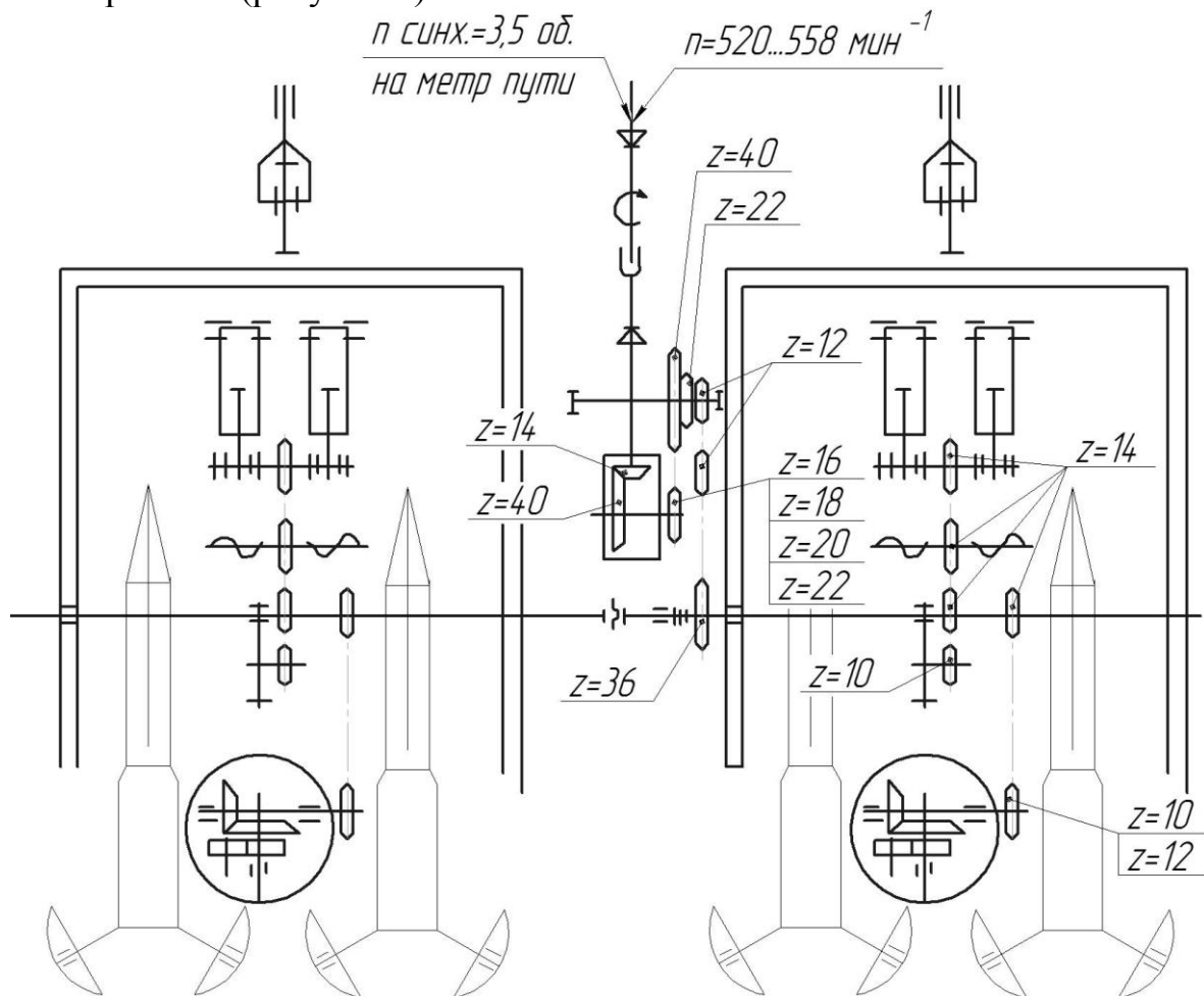
Рисунок 2 – Кинематическая схема привода сажалки СН-4Б
