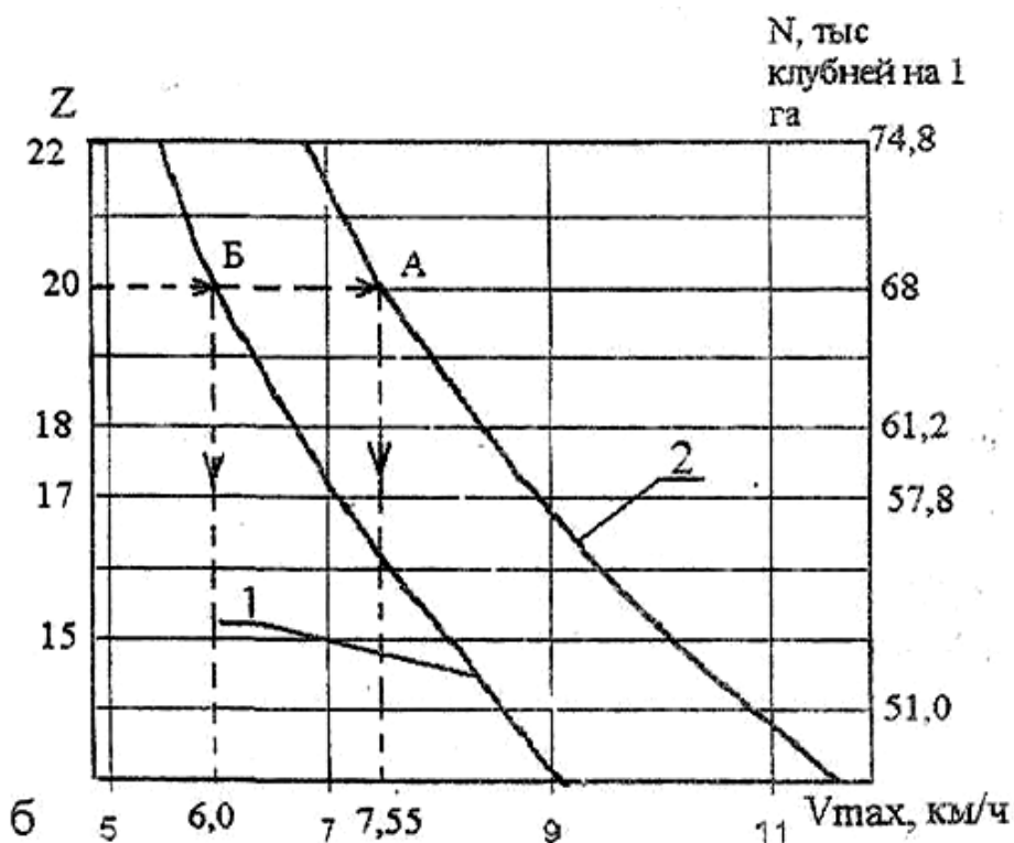
Рисунок 6 - Номограммы для предварительного выбора режимов работы при синхронном приводе 13,15,17,18,20,22 - сменные звездочки с соответствующим числом зубьев, 1 - большие ложечки для клубней 80...120 г, 2 - основные ложечки для клубней 25...80 г.
