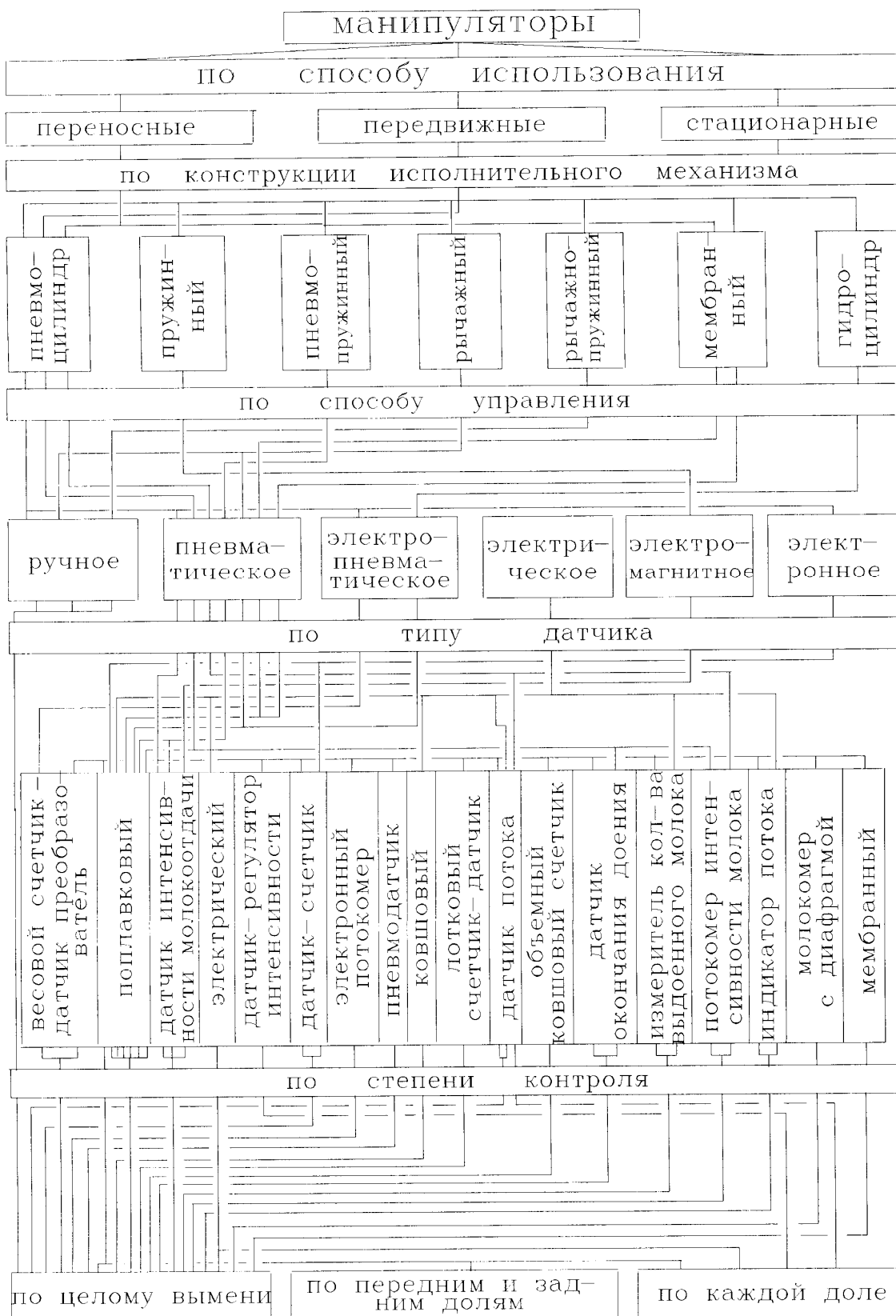
Рисунок 1.7 - Классификация манипуляторов доильных установок по способу использования и конструкции исполнительных механизмов
