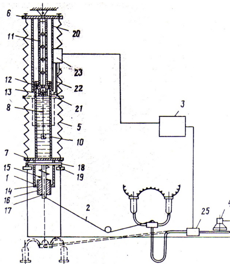
Рисунок 1.1 - Схема устройства для снятия доильного аппарата
