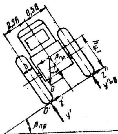
Рисунок 3.4 – Схема к определению устойчивости трактора
