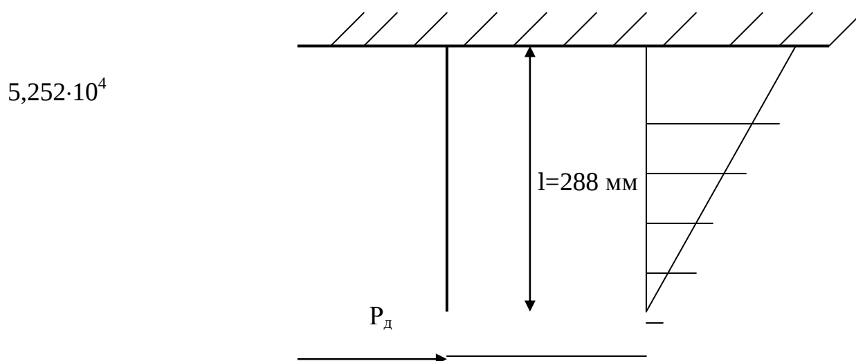
Рисунок 3.1 - Схема по определению нагруженности зуба гребёнки
