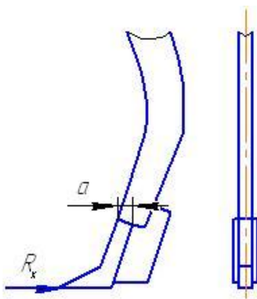
Рисунок 3.2 – Расчётная схема
