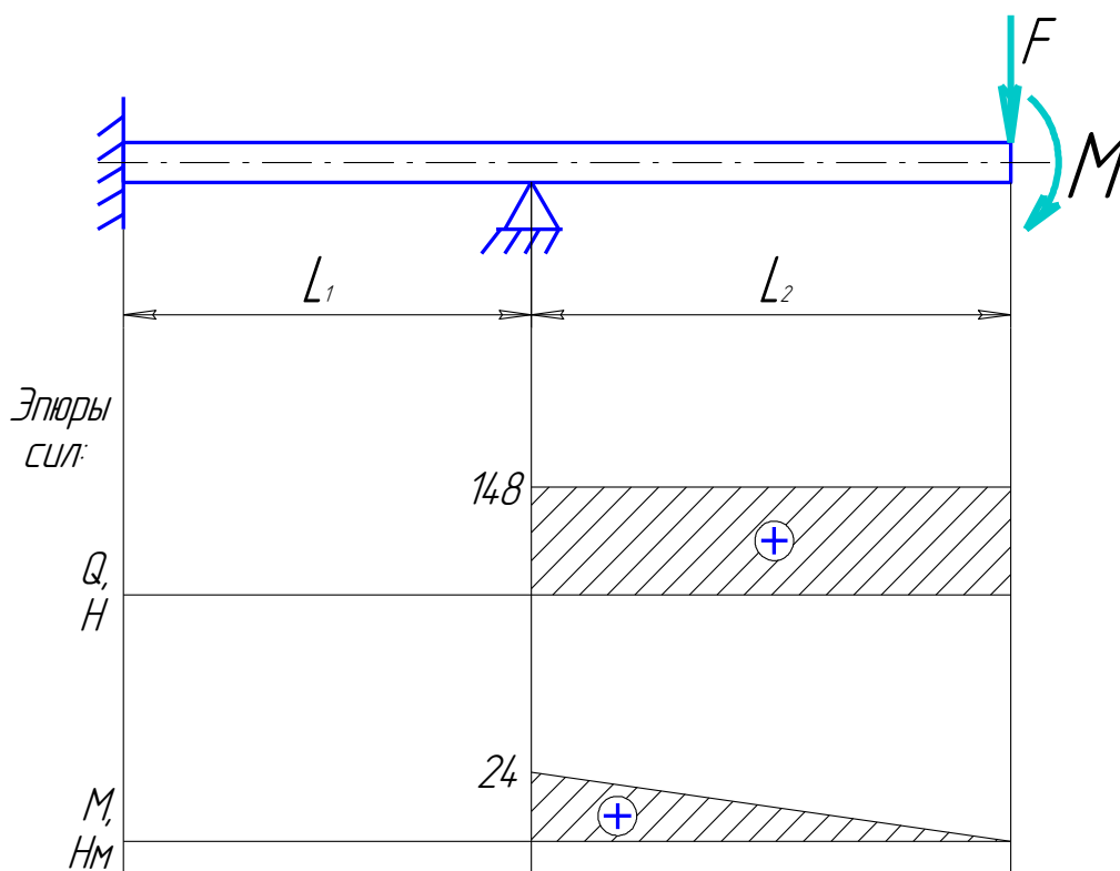
Рисунок 3.3 Расчетная схема
