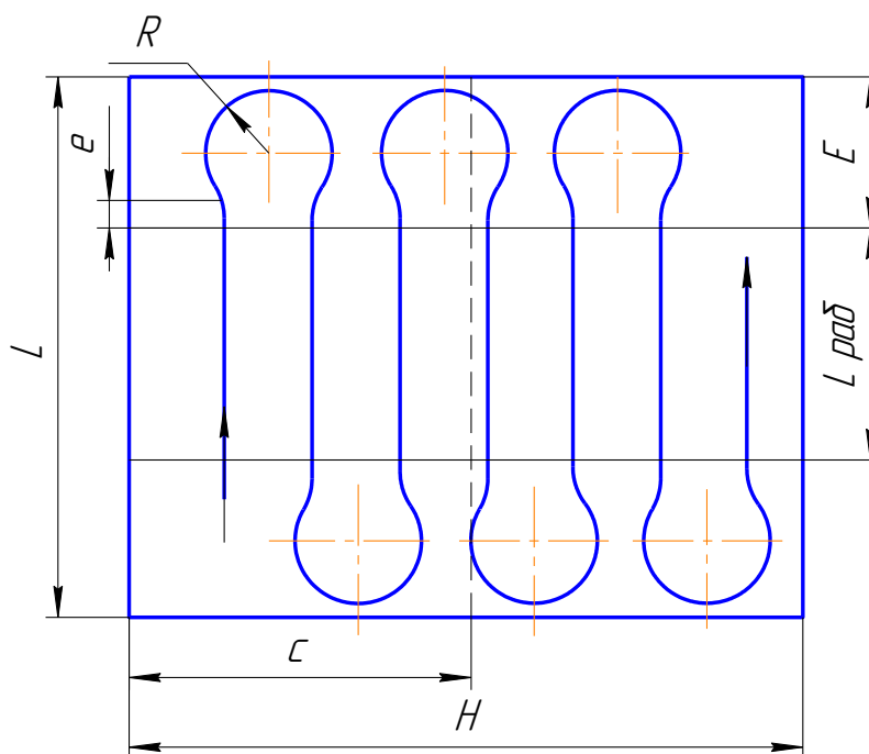
Рисунок 2.1 – Схема движения агрегата по полю
