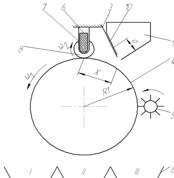
Рисунок 1.4 - Диэлектрический сепаратор (АС СССР № 1450867)
