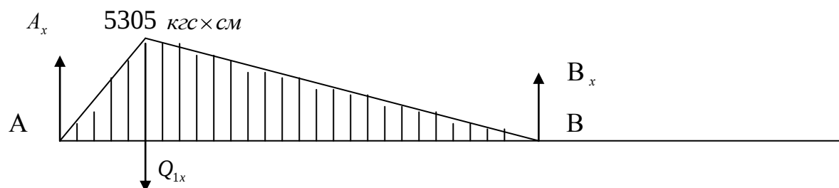
Рисунок 3.6- Эпюра изгибающего момента
