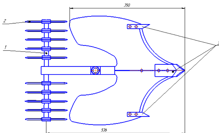
Рисунок 3.2-Рабочий орган культиватора-плоскореза
