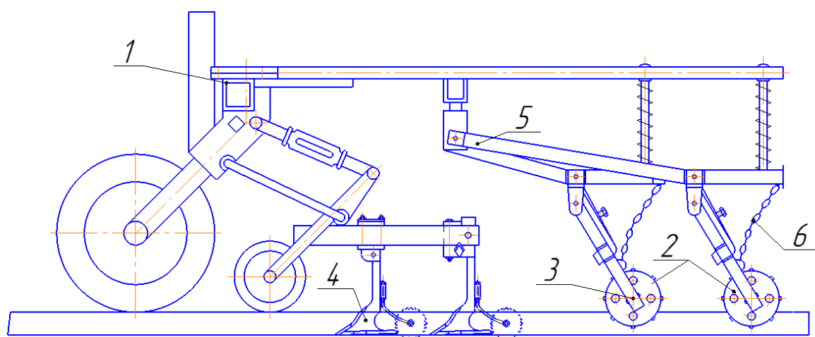
Рисунок 3.1 – Почвообрабатывающая машина
