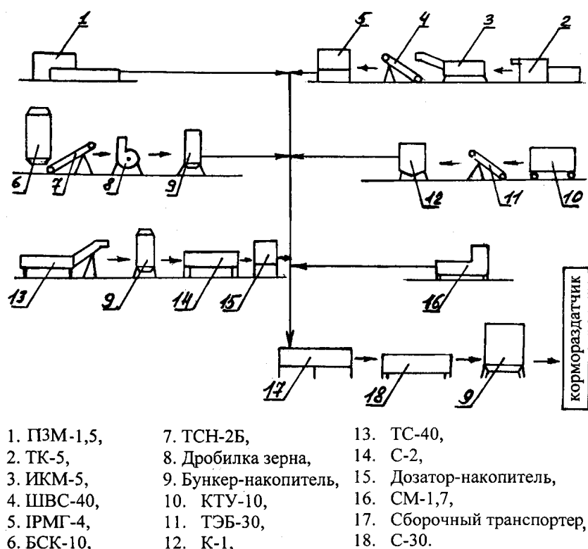
Рисунок 1.3 – Схема технологического процесса кормоцеха третьего типа
