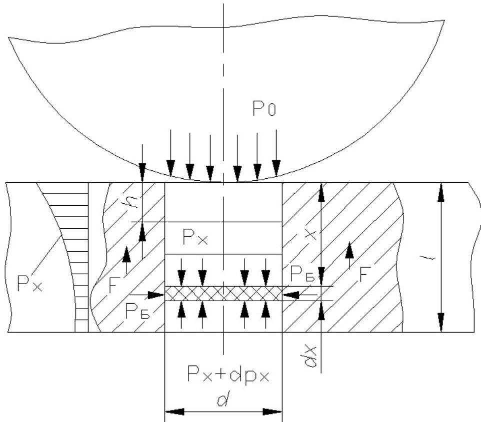
Рисунок 3.4 – Расчетная схема узла прессования с плоской матрицей
