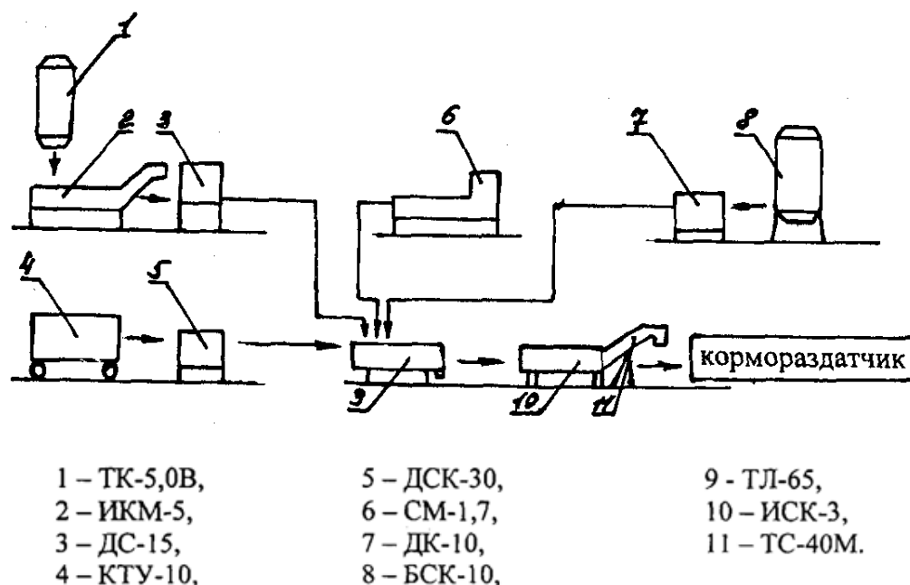
Рисунок 1.1 - Схема технологического процесса кормоцеха первого типа
