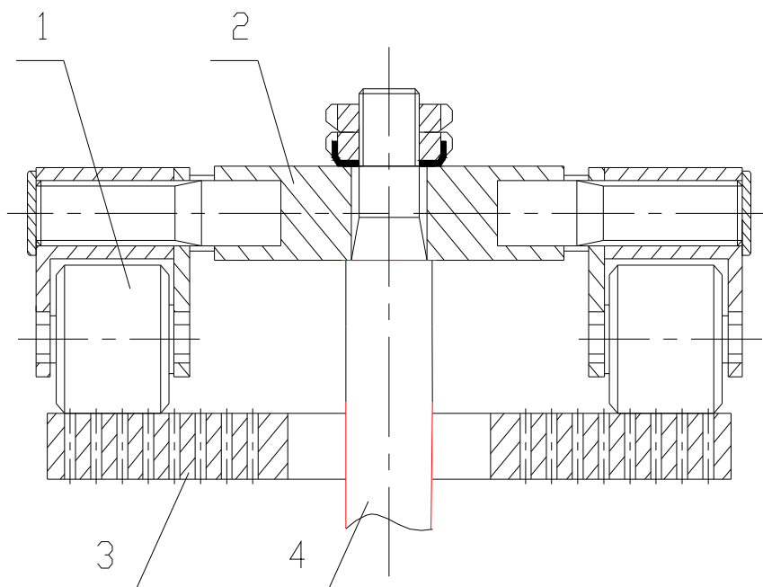
1 – прессующие вальцы; 2 – водило; 3 – матрица; 4 – вал Рисунок 3.3– Принципиальная схема узла прессования с плоской матрицей
