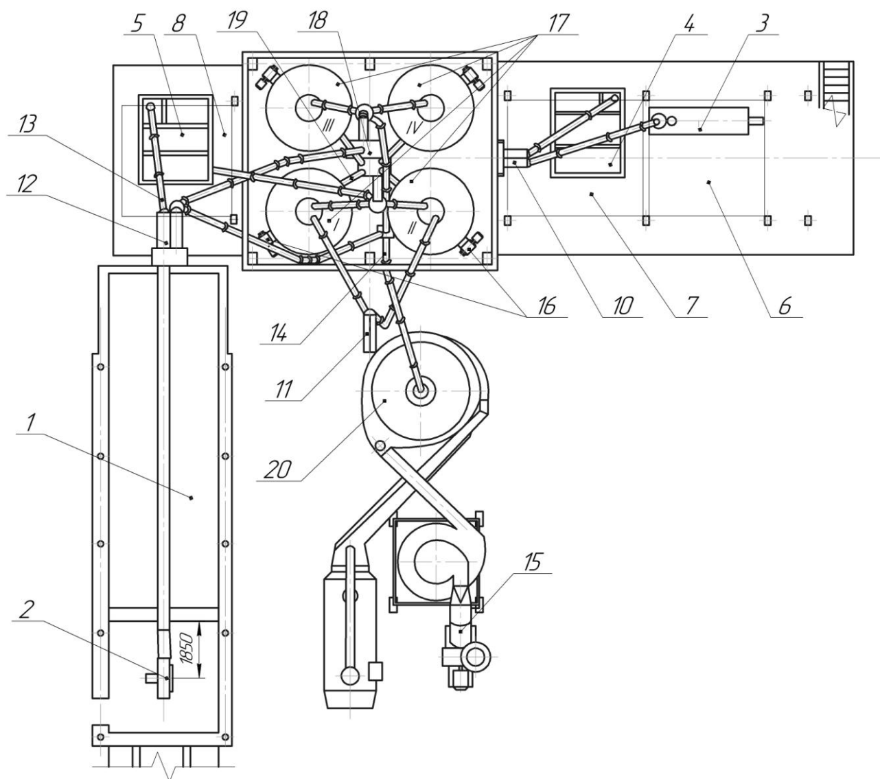
Рисунок 2.1 – Технологическая схема предлагаемого зерносушильного комплекса
