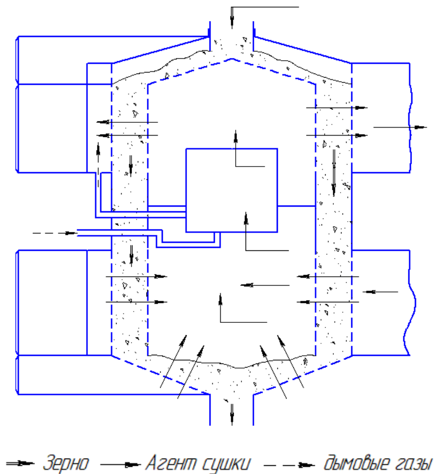
Рисунок 3.2 – Расчетная схема зерносушилki
