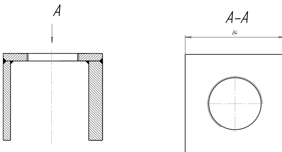
Рисунок 3.5.4 - Сварное соединение корпуса двигателя
