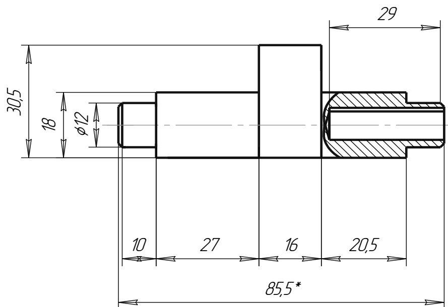
Рисунок 3.5.1 - Кулачковый вал
