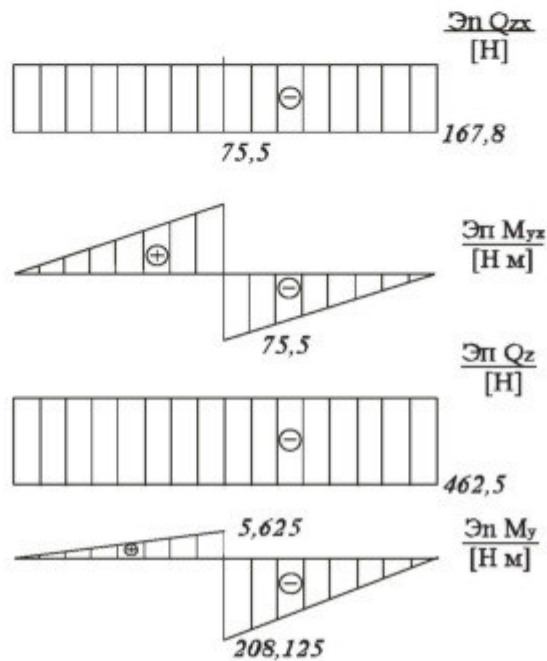
Рисунок 3.2 - Эторы поперечной силы и изгибающего момента.
