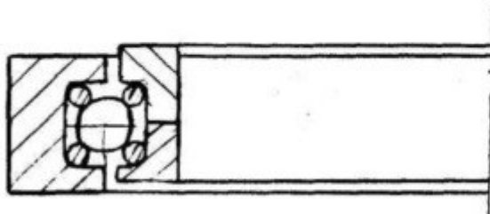
Рисунок 3.3 - Схема поворотного подшипника
