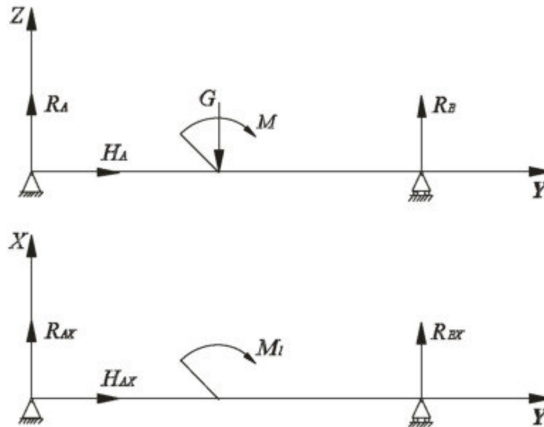
Рисунок 3.1 - Схема нагружения направляющей.
