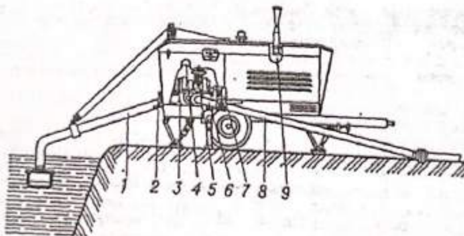
Рисунок 11. - насосная станция ДНУ- 120/70
